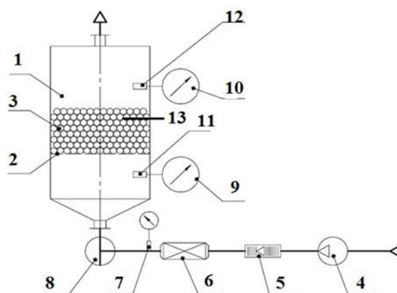
Рисунок 3 – Схема экспериментальной установки конвективной сушки 1 – корпус сушки, 2 – опорная решетка, 3 – початки рогоза, 4 – воздуходувка, 5 – ротаметр, 6 – калорифер, 7 – термометр, 8 – кран шаровой, 9, 10 – термогигрометры, 11, 12 – датчики термогигрометров, 13 – термометр.
