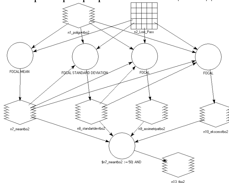
Рисунок 4 - Общая модель для выявления свалки отходов на космическом снимке
