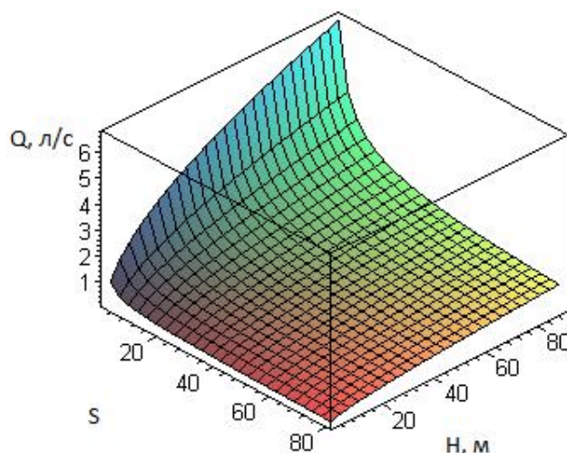
Рисунок 1 – Зависимость расхода воды из ПКК от свободного напора H=(2 \div 90) м и сопротивления ПКК S=(2 \div 80)
