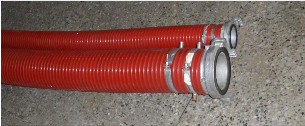
Фото № 1 - Вид шлангов спиральных армированных из ПВХ
